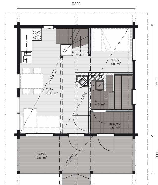
Hukkanen 43 P Vaihtoehtoinen pohjapiirros (parvellinen) Alternativ planritning (med loft)
