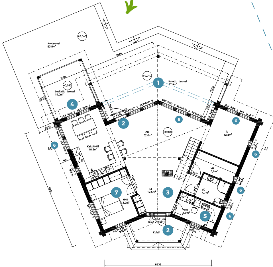
Nuuna 205 T2 1. krs. pohjapiirros. Nuuna 205 T2, planritning för bottenplan
