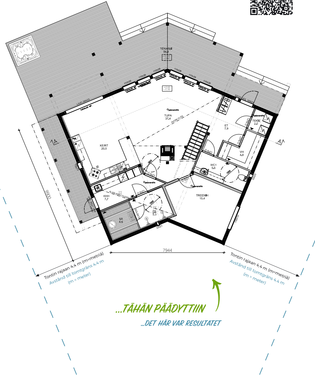
Nuuna 205 T2-muunnoksen 1. krs. pohjapiirros. Nuuna 205 T2-variant, planritning för bottenplan
