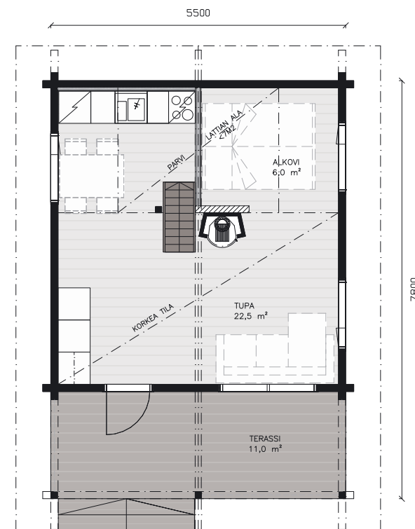
Hannus 32 P Vaihtoehtoinen pohjapiirros (parvellinen) Alternativ planritning (med loft)
