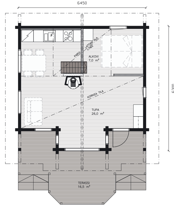
Vaihtoehtoinen pohjapiirros (parvellinen) Alternativ planritning (med loft)
